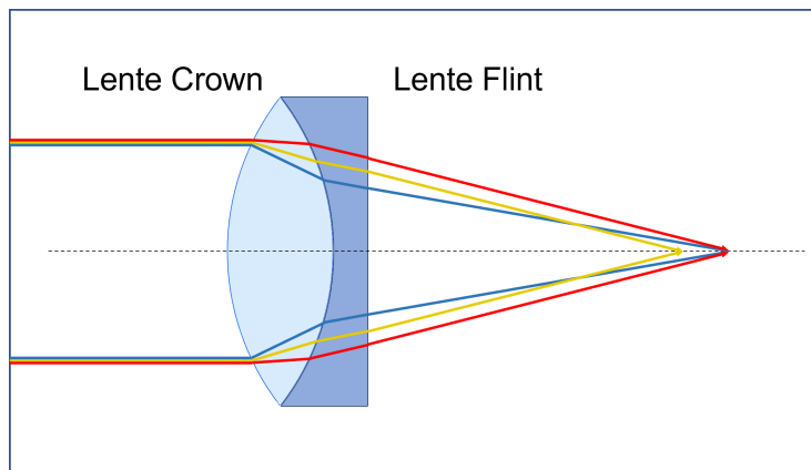
Figura 2: Representação esquemática de uma lente dupla. Na imagem, a montagem é a de Fraunhofer, na qual a lente Flint é plano-côncava e encaixa perfeitamente na lente Crown.
