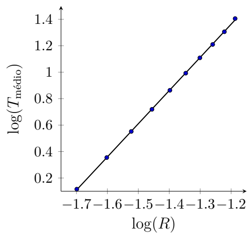
Gráfico 1: \log(T_{\text{médio}}) x \log(R)
