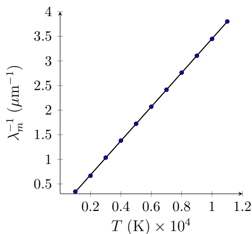
Gráfico 2: Temperatura ( T ) x Inverso do comprimento de onda máximo ( \lambda_m^{-1} )
