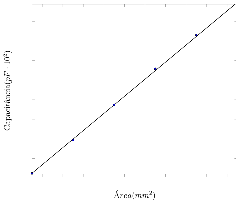
Gráfico 1.1: Área vs Capacitância(Mica)
