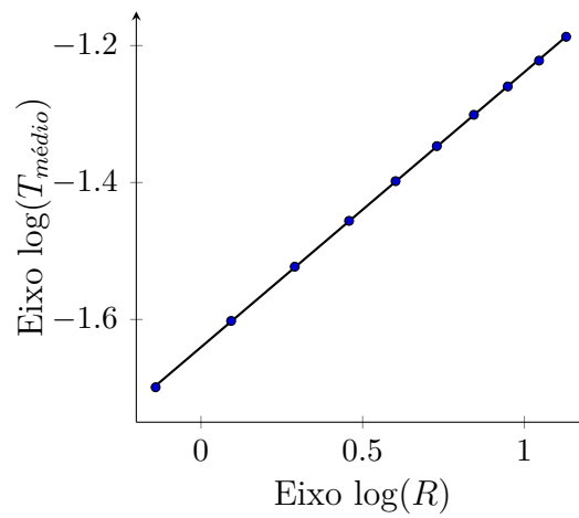
Gráfico 2: dados linearizados
