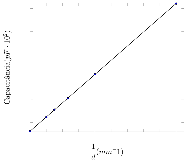
Gráfico 2: Inverso da Distância vs Capacitância(Papel)
