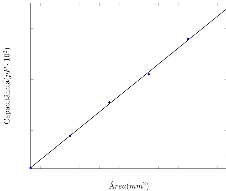
Gráfico 1.2: Área vs Capacitância(Papél)
