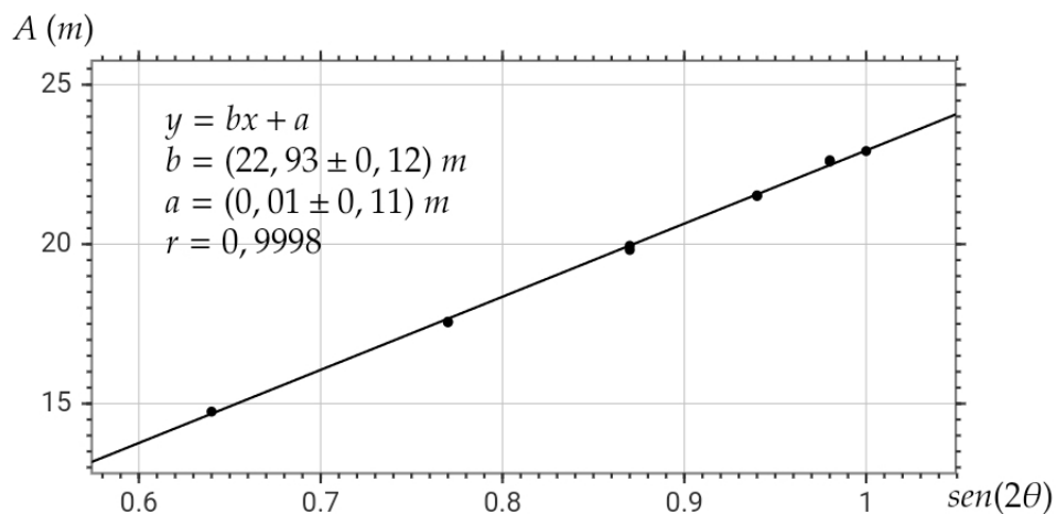
Gráfico 01 : A (m) por \operatorname{sen}(2\theta)
