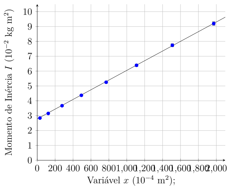
Gráfico 2.2: I_3 \times d_3
