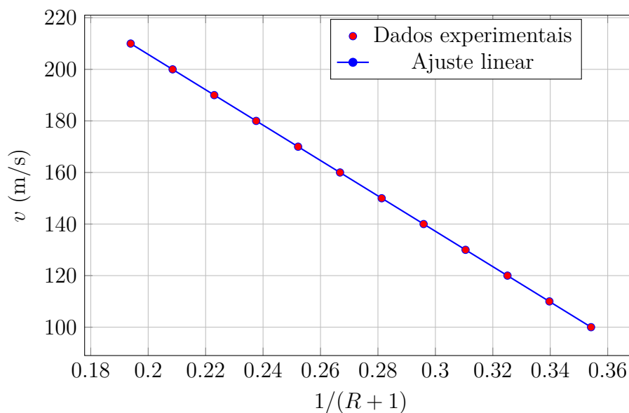
Gráfico v vs 1/(R+1)
