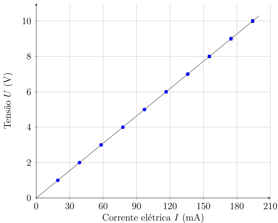
Gráfico 1.3: U vs I para R_6
