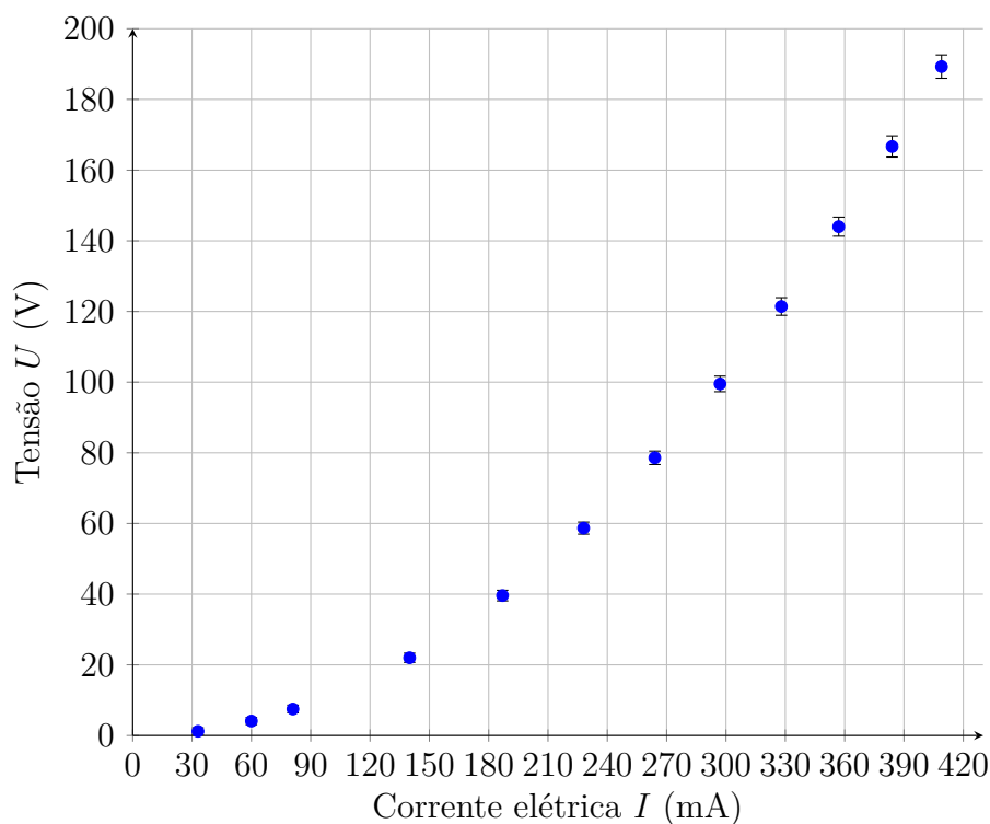
Gráfico 2: Curva U vs I para L_1
