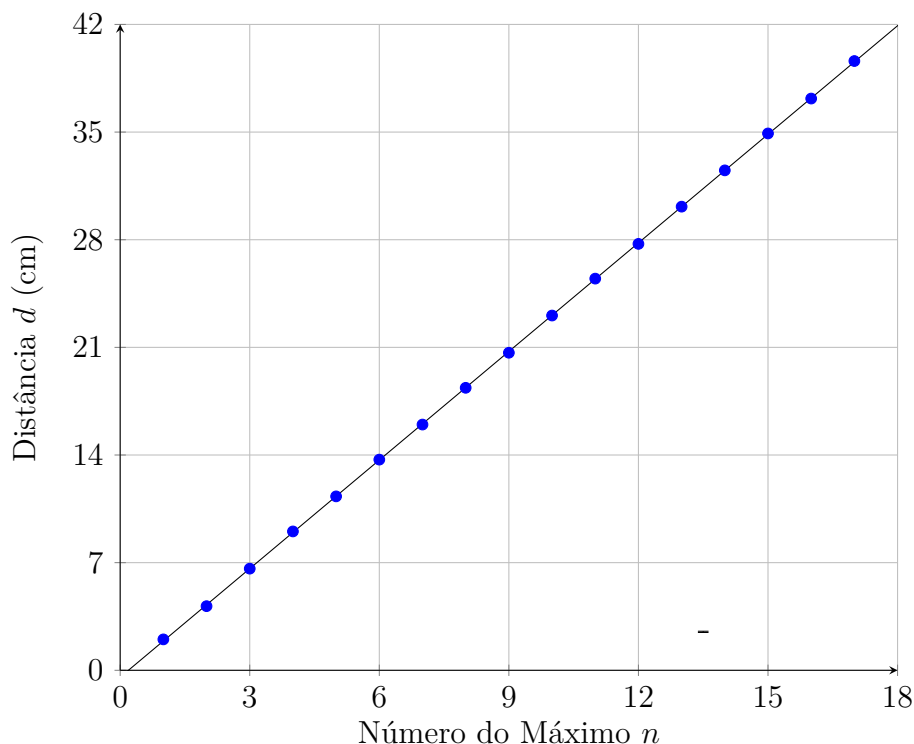
Gráfico 1.1: d vs n para \lambda_1
