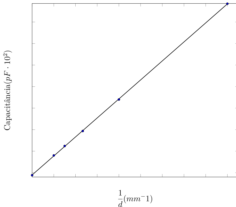
Gráfico 1: Inverso da Distância vs Capacitância(Mica)
