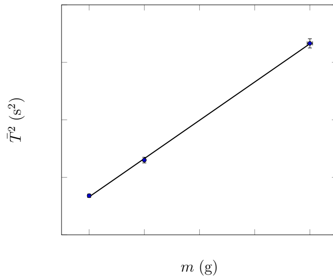
Gráfico 1: Período para cada massa
