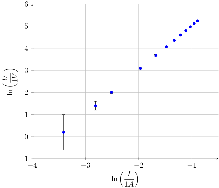
Gráfico 3: Curva linearizada \ln U vs \ln I para L_1
