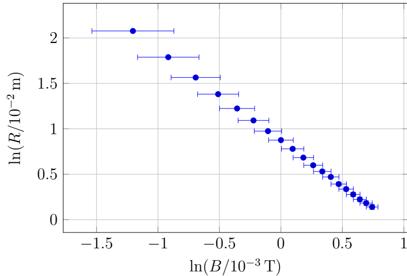
Gráfico 3: Dependência linearizada entre B e R
