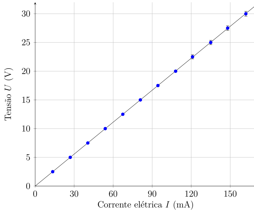
Gráfico 1.1: U vs I para R_1
