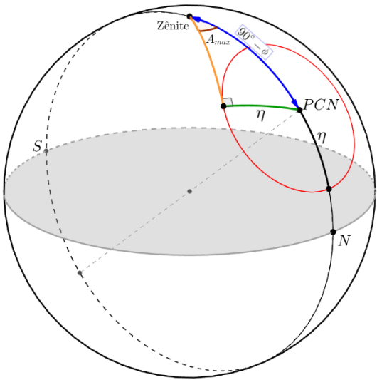
Figura 5.55: Azimute máximo
