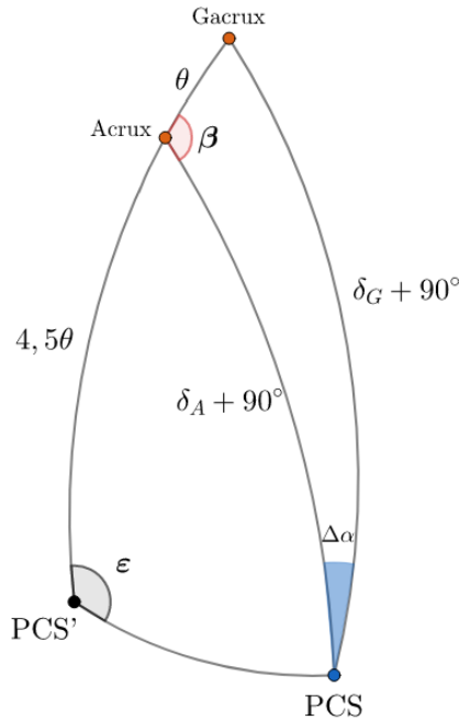
Figura 5.53: Triângulos esféricos da situação
