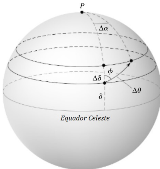
Figura F.5: Movimento próprio na esfera celeste
