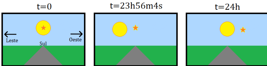
Figura 6.14: Consequência da diferença entre o dia sidereal e o dia solar
