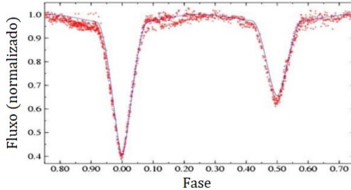
Figura 7.30: Fluxo normalizado
