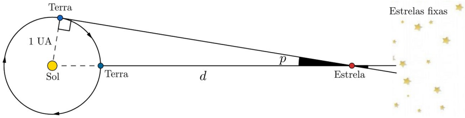
Figura B.4: Paralaxe heliocêntrica
