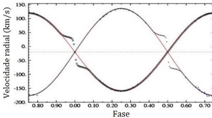
Figura 7.31: Velocidade radial
