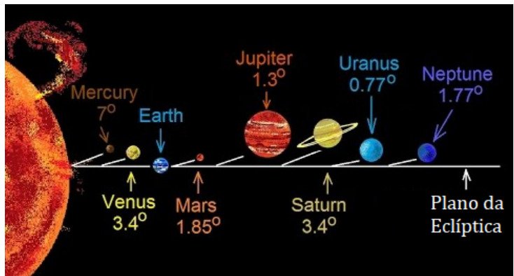
Figura C.3: Inclinação da órbita
