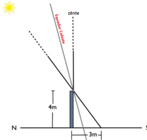
Figura 5.43: O poste e sua sombra
