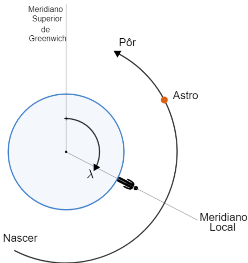
Figura 6.3: Movimento diário dos astros
