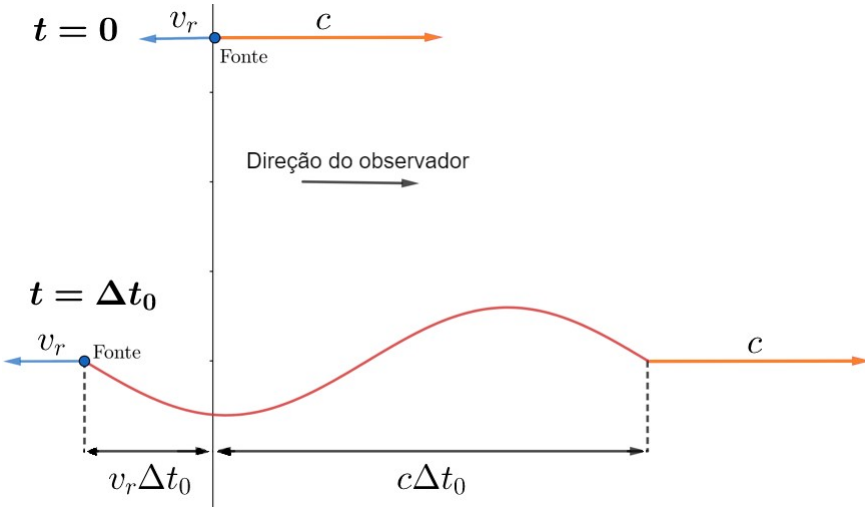
Figura 3.8: Redshift
