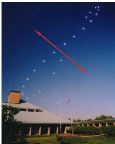
Figura 6.4: Analema
