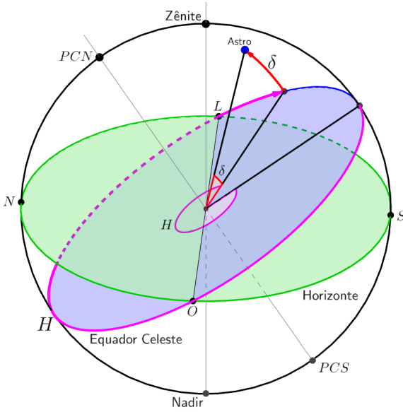
Figura 5.12: Primeira convenção
