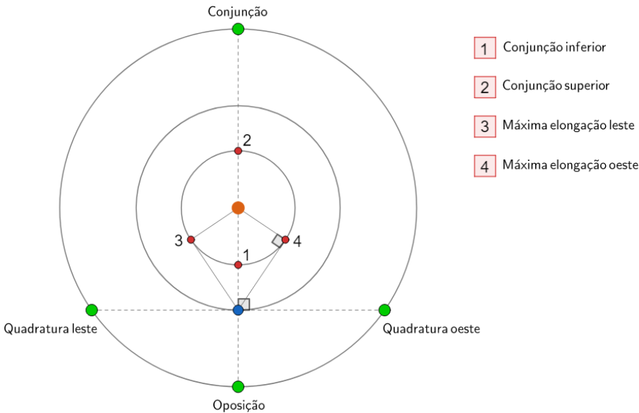
Figura C.9: Configurações Planetárias
