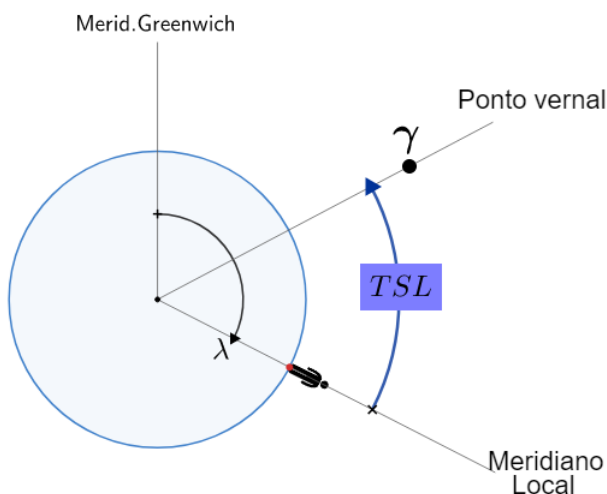
Figura 6.15: TSL
